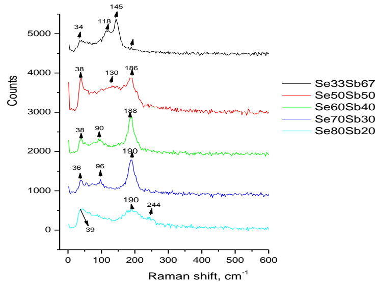
Şəkil 2. XŞY Se –Sb sisteminin raman səpilmə spektri
