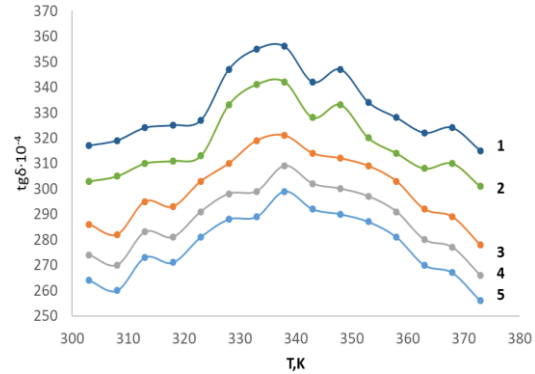
Şəkil 1. ASPE= x həcm% BP+ y həcm% Fe tip nanokompozitlərinin dielektrik nüfuzluqlarının (a) və dielektrik itki bucaqlarının (b) temperatur asılılıqları: 1-x=1; 2-x=3; 3-x=5; 4-x=10; 5-x=15.
