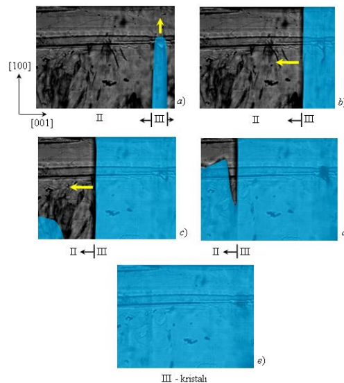
Şəkil 2. K_{0,940}Ag_{0,060}NO_3 kristalında II \rightarrow III çevrilməsi zamanı III modifikasiya kristalının böyümə morfolojiyasını əks etdirən mikrofotografiyalar (Böyütmə \times 90 dəfə). Foto e) III-modifikasiya kristalı tam II \rightarrow III çevrilmədən sonra.
