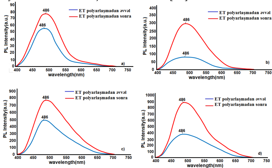
Şəkil1. PP+SiO 2 əsaslı polimer nanokompozitlərin fotolüminessensiya spektrləri a)PP+1%SiO 2 b) PP+3%SiO 2 c) PP+5%SiO 2 d) PP+7%SiO 2
