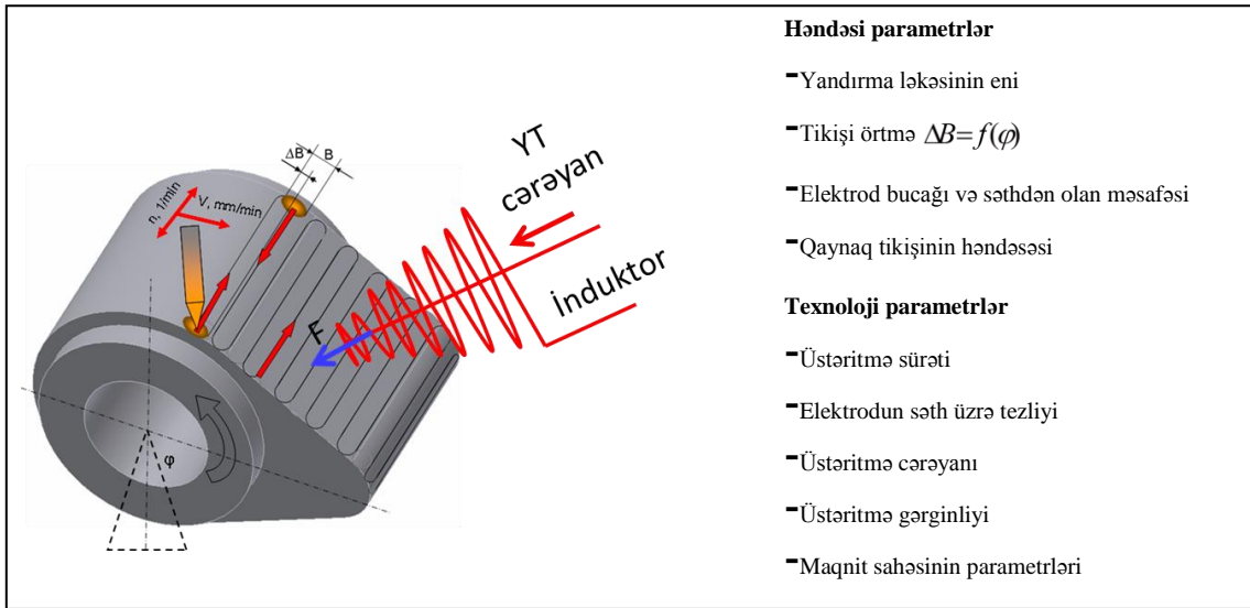
Şəkil 1. Yüksək tezlikli maqnit sahəsində yuzamanı induktorla detalın qarşılıqlı vəziyyəti, yandırma ləkəsinin səth üzrə hərəkət sxemi, həndəsi və texnoloji parametrlər.
