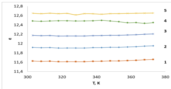
Şəkil 1. ASPE= x həcm% BP+ y həcm% Fe tip nanokompozitlərinin dielektrik nüfuzluqlarının (a) və dielektrik itki bucaqlarının (b) temperatur asılılıqları: 1-x=1; 2-x=3; 3-x=5; 4-x=10; 5-x=15.
