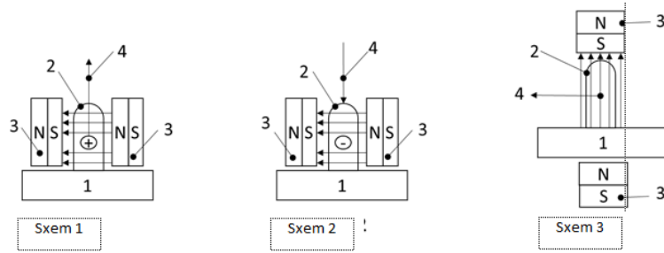
Şəkil 1. Sabit maqnitlərin və əlavə cərəyanın tətbiqi ilə əridilmiş materiala formanın verilməsi.
