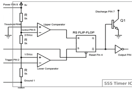
Şəkil 1. NE555 mikrosxeminin daxili strukturu
