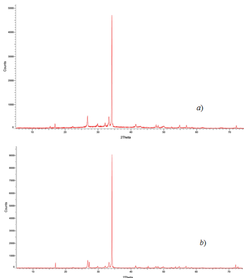
Şəkil 1. GeS monokristalının difraktoqrammaları. a) şüalanmaya qədər; b) 50 krad şüalanmadan sonra.
