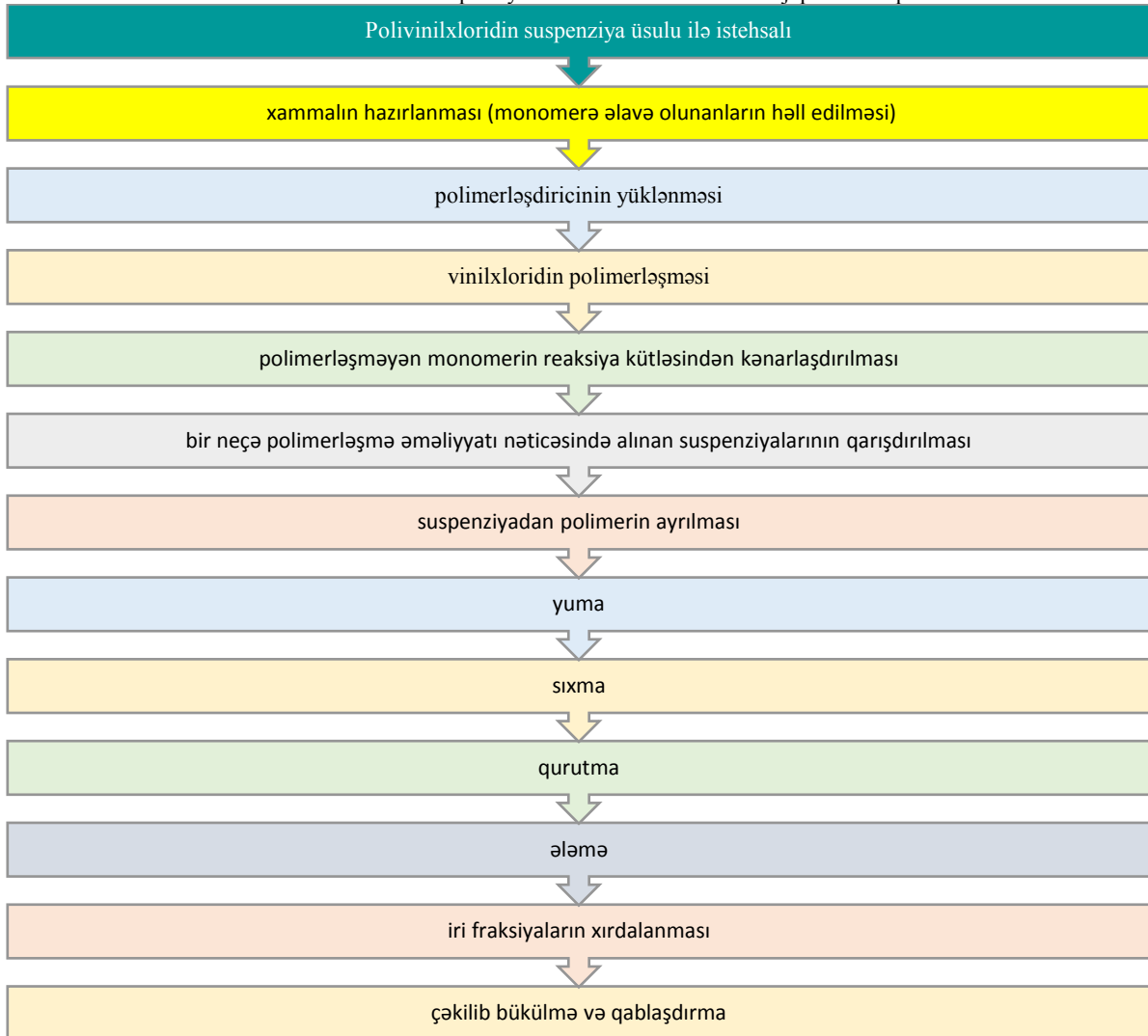
Cədvəl1. Polivinilxloridin suspenziya üsulu ilə istehsalının texnoloji prosesinin pillələri
