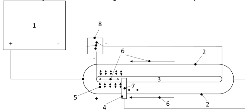
Şəkil 2. Sabit maqnit induktorlarının və cərəyanın tətbiqi ilə maye metala formanın verilməsi.
