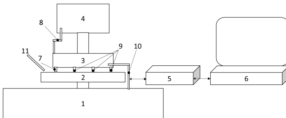
Şəkil 1. Paradaqlama-cilalama maşını bazasında tribotexniki sınaq qurğusu
