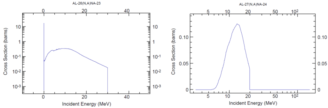
Şəkil 1. Neytron selinin Al fərqli izotoplarında yaratdığı (n, α) çevrilmələrinin effektiv en kəsiyi spektrləri.
