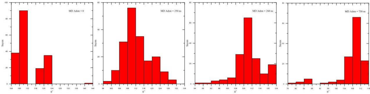
Şekil 3. Simülasyon adım sayısına göre \Theta açısı değerleri
