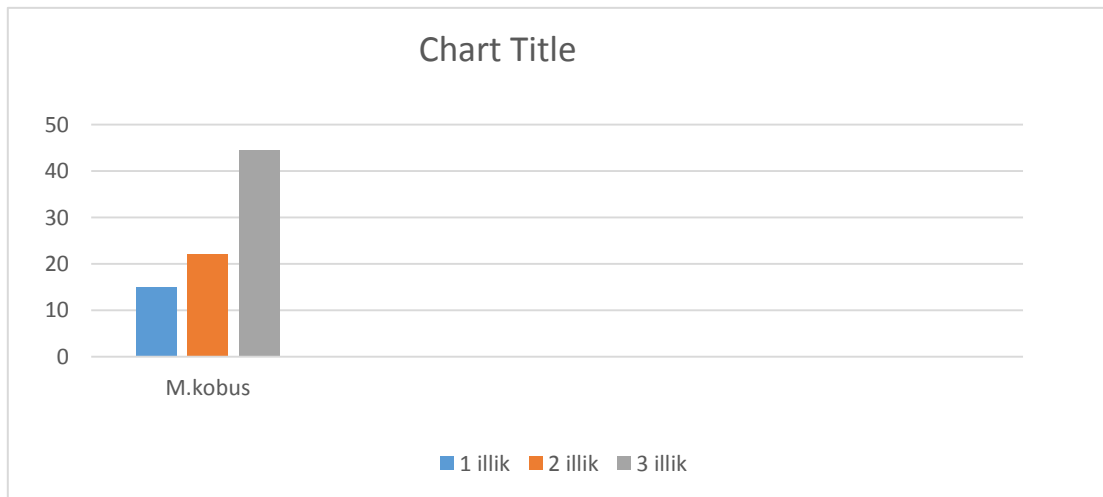
Diaq.1. Tədqiq olunan M.kobus növünün 1-3 illik tinglərinin hündürlüyü
