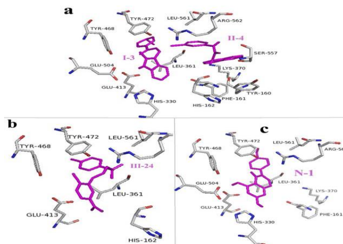
Şəkil 1. I-3, II-4 (a), III-24 (b) və N-1 (c) inhibitorlarının bakterial qlükuronidazanın fəal mərkəzi ilə molekulyar dokinqi
