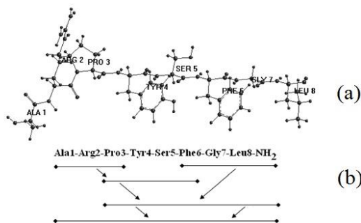
Şəkil 1. DİPPU AST6 allatostatin molekulunun fəza quruluşu (a) və hesablama sxemi (b)
