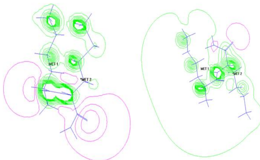
Şəkil 1. L-Met–L-Met dipeptidinin enerji cəhətdən ən əlverişli konformasiyalarının R 22 R 32 (a) və B 21 B 21 (b) elektron sıxlığı.
