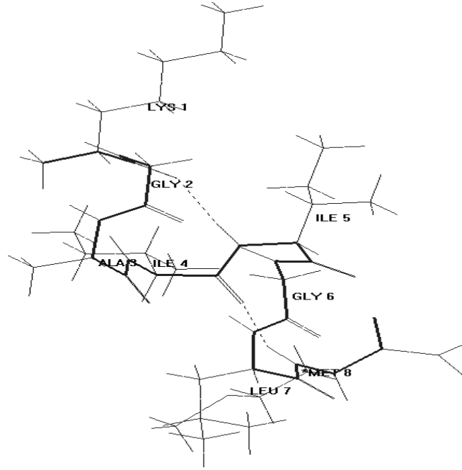
Şəkil. 2. A \beta (28-35) peptidinin enerji cəhətdən ən əlverişli konformasiya (R 22 RR 12 R 32 R 32 RR 21 R 32 )
