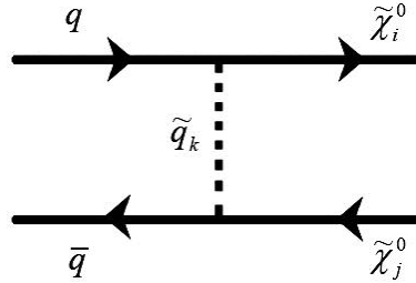
Рис.3 Диаграмма Фейнмана для t -канала подпроцесса столкновения двух кварков а) t - канал без поляризации
