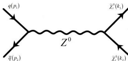
Рис.2 Диаграммы Фейнмана процесса рождения пары нейтралино при столкновении протонов с высокими энергиями с участием виртуального Z^0 бозона
