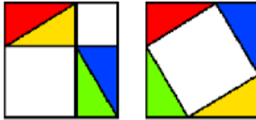
Şəkil 1. Pifaqor Teoreminin Sözsüz İsbatı
