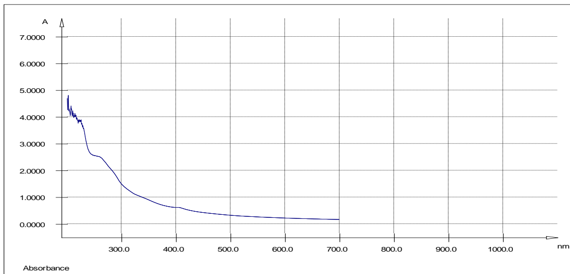
Şəkil 2. UV – VİS spektrofotometrik analiz, Broth qidalı mühitdə 400-450 nm udulma halı
