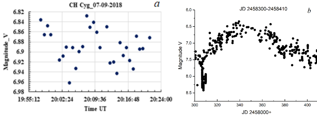
Şəkil 1. CH Cyg-nin V filtrində parlaqlıq əyrisi. a - 07-09-2018, b - 30-06 ÷ 18-10-2018.
