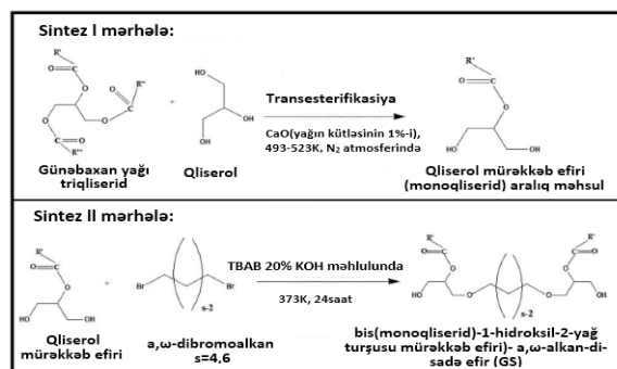
Şəkil1. Günəbaxan yağından 2 mərhələdə neytral ikili səthi aktiv maddə (GS) sintezi reaksiyaları.
