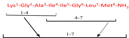
Şəkil 1. Aβ (28-35) peptidin optimal uyğunluğunun hesablanması sxemi
