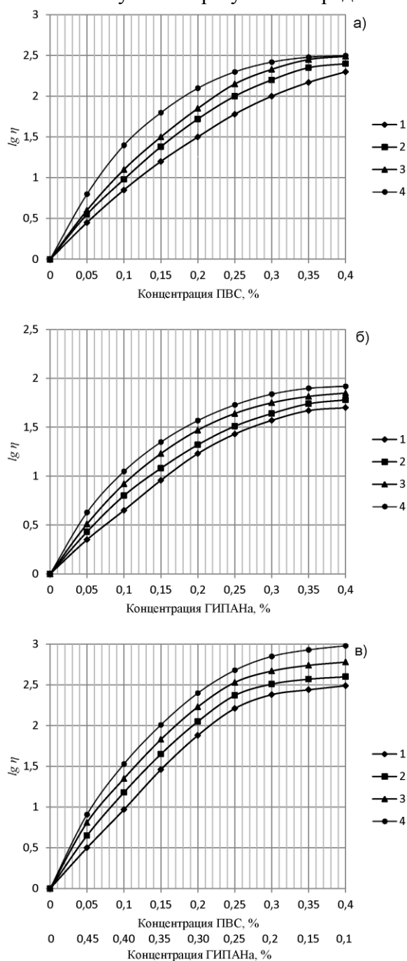
Рис. Зависимость вязкости шлихтующих композиций от содержания в них ПВС (а), ГИПАНа (б) и при совместном присутствии ПВС и ГИПАНа (в), концентрации крахмала, %:
