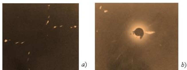
Şəkil 4. K_{0,940}Ag_{0,060}NO_3 kristalında \text{II} \rightarrow \text{III} çevrilmədən əvvəl (a) və sonra (b) çəkilən laueqramlar.
