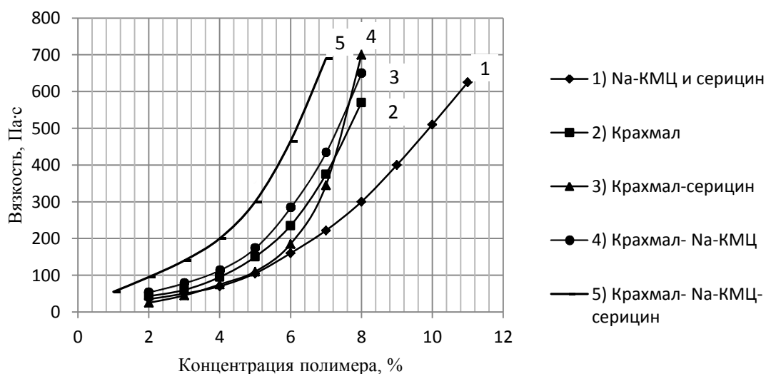
Рисунок. Зависимость вязкости гелеобразных загусток от концентрации компонентов загущающих ингредиентов и времени выдерживания
