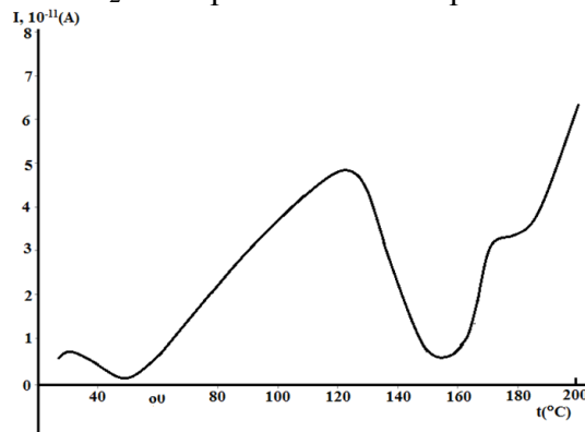
Şəkil2. PP+3%SiO 2 əsaslı polimer nanokompozitlərin TSD spektri
