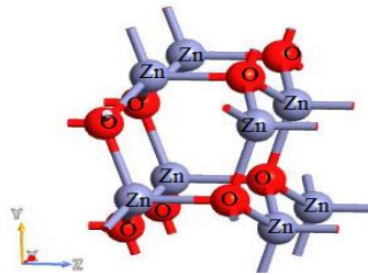
Şəkil. ZnO-nunkristal quruluşu.
