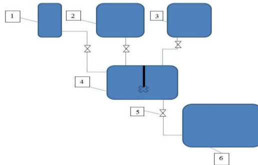
Şəkil 1. Quyudibi zonanın keçiriciliyinin artırılmasına imkan verən nanosistemin hazırlanmasının texnoloji sxemi
