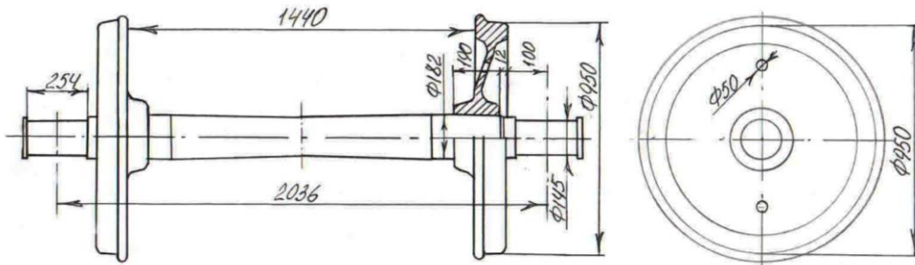
Şəkil 1. 10507-H yığma cizgisində təkər cütünün 10509-H tam döyülmüş təkərinin işçi cizgisi.
