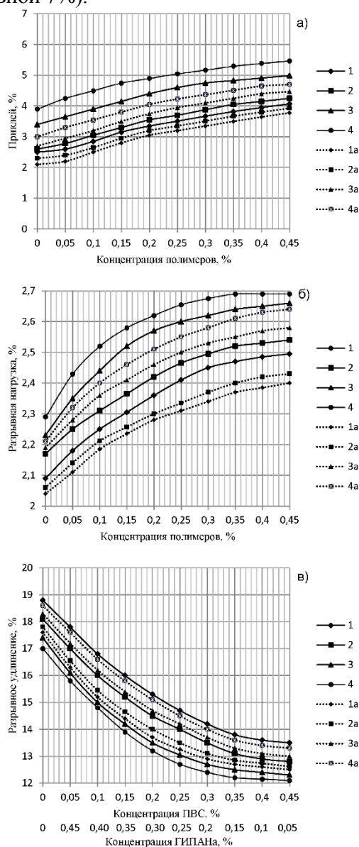
Рис. Влияние концентрации ПВС и ГИПАНа в шлихтующем составе на параметры ошлихтованной пряжи Концентрация крахмала, %: 1-4; 2-4,5; 3-5; 4-5,5 (1а, 2а, 3а, 4а – крахмальная шлихта без ПВС и ГИПАНа)
