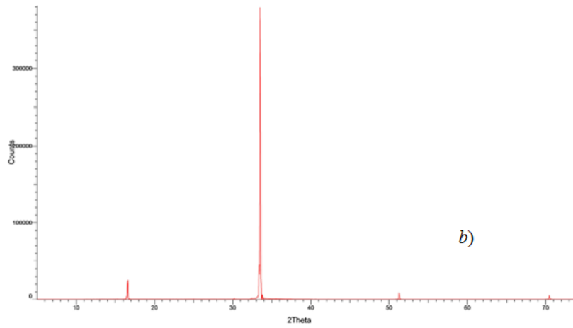
Şəkil 2. \text{Ge}_{0.995}\text{Er}_{0.005}\text{S} kristalının difraktoqramları. a) şüalanmadan əvvəl; b) 50 krad şüalanmadan sonra.
