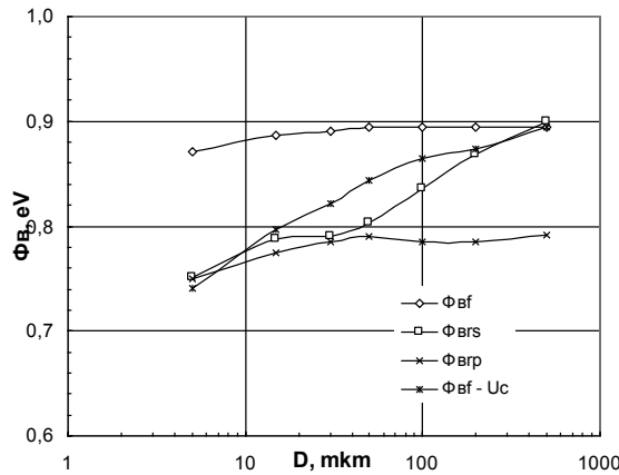
Şəkil 1. Au-nGaAs Şotki diodlarının potensial çəpərinin \Phi_{Bf} , \Phi_{BrP} və \Phi_{BrS} hündürlüklərinin və ( \Phi_{Bf} - U_c ) fərqi-nin kontakt diametrindən asılılıqları.
