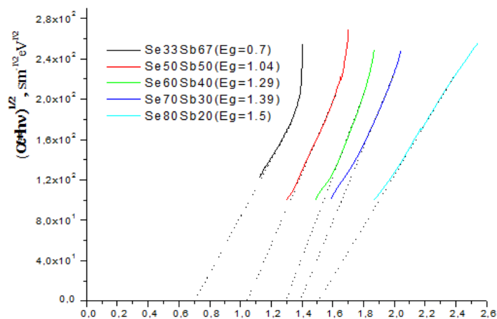
Şəkil 1. XŞY Se – Sb sisteminin optik udma spektrləri.
