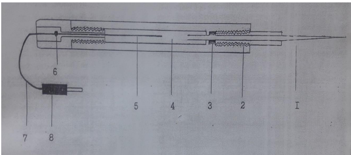
Şəkil 1. Mikroelektrod holderi. İdarələr: 1- mikroelektrod, 2 – sıxıcı qayqa, 3 – rezin kipləşdirici, 4 – doymuş KCl və ya 1M NH 4 Cl məhlulu ilə doldurulmuş fəza, 5 – Ag – AgCl elektrodu, 6 - Ag – AgCl elektrodunun birləşdirici naqillə lehim yeri, 7 - birləşdirici naqıl, 8 – ölçü cihazları ilə birləşdirən ştekker.
