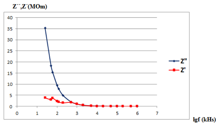
Şəkil 1. YSPE+10% PKR-3M kompozit nümunələri üçün Z''(1) və Z'(2) tezlik asılılığı
