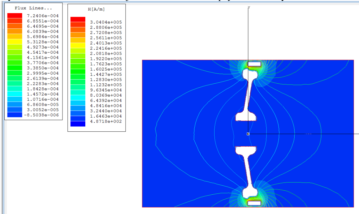
Şəkil 3. Hesablanmış maqnit sahəsinin vizuallaşdırılması.
