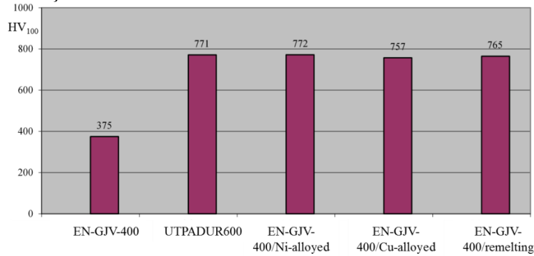
Şəkil 2. Yumruq üzərinə çəkilmiş təbəqənin bərklik diaqramı
