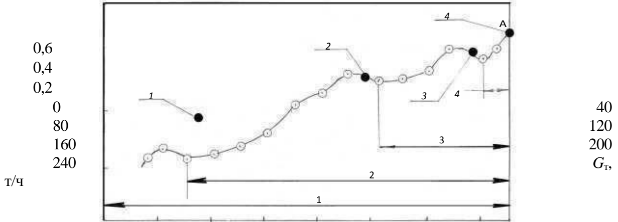
Şəkil 2. İdarəetmə mərhələsinin daxili səmərəliliyinin tur turbindəki buxar axınının sürətindən asılılığı: - çökmə rejimləri, - klapanlar tamamilə açıqdır
