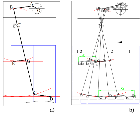
Şək. 1. Bir tərəfə (a) və iki tərəfə (b) açılan ikitaylı qapı mexanizminin struktur sxemi.
