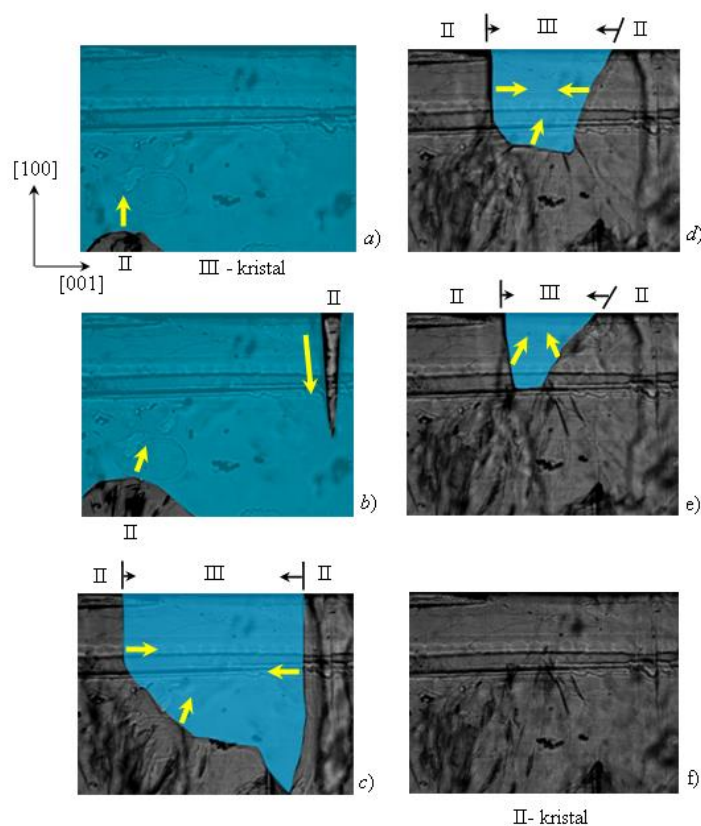
Şəkil 3. K_{0,940}Ag_{0,060}NO_3 kristalında \text{III} \rightarrow \text{II} çevrilməsi zamanı II modifikasiya kristalının böyümə morfolojiyasını əks etdirən mikrofotoqrafiyalar (Böyütmə \times 90 dəfə).
