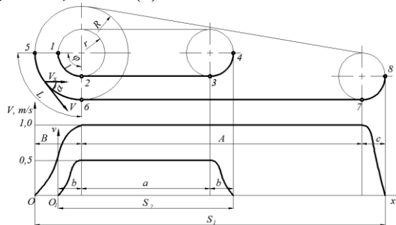
Şək. 3. Elastik intiqallı ikitaylı lift qapısının hərəkət sürətinin onların gedişindən asılılıq qrafiki.
