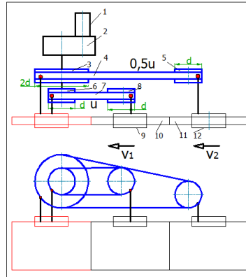
Şək. 2. İkitaylı qapı mexanizminin yeni konstruktiv həlii.
