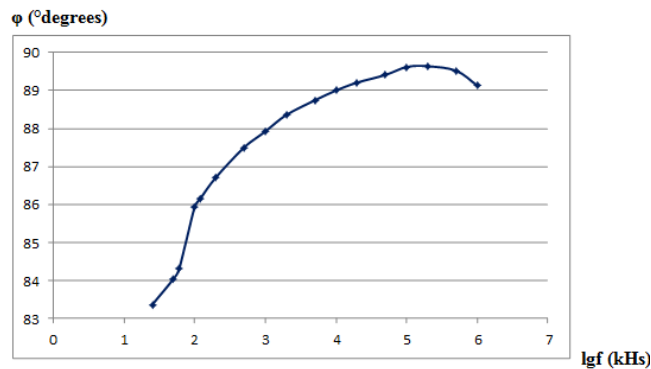
Şəkil 2. YSPE+10% PKR-3M kompozit nümunələri üçün \varphi bucağının tezlikdən ( lgf ) asılılığı qrafiki
