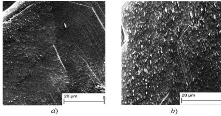
Şəkil 3. GeS laylı monokristalının səth morfologiyası. a) şüalanmadan əvvəl; b) 50 krad şüalanmadan sonra
