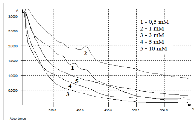
Şəkil 3. Saccharomyces ellipsoideus BDU – XRI ştamının gümüş nitratın qatılığında asılı olaraq biokütlədə əmələ gətirdiyi gümüş nanohissəciklərin UV- spektrləri
