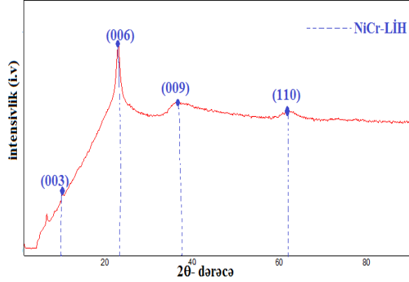
Şəkil1. NiCr-laylı ikili hidroksidin RD analizi
