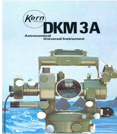
Şəkil 1. Kern DKM 3-A Universal teodoliti
