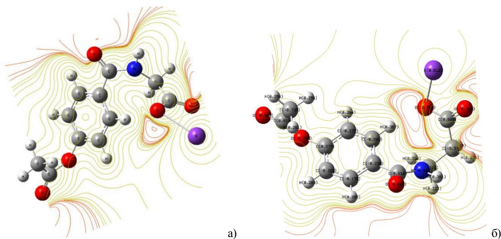
Рис.1. 3D структура, распределение зарядов и электронной плотности: а) N-(4-ацетоксибензоил)глицинат калия и б) 4-[(N-4-ацетоксибензоил)амино]бутанат калия
