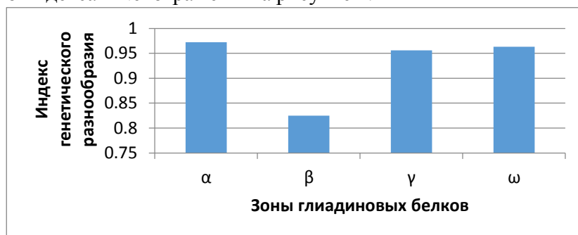
Рис.2. Индексы генетического разнообразия, подсчитанные по зонам глиадиновых белков.
