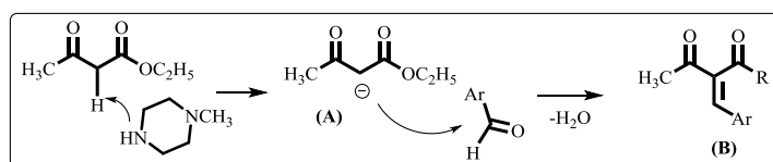
Схема 1. Конденсация Кневенагеля.
