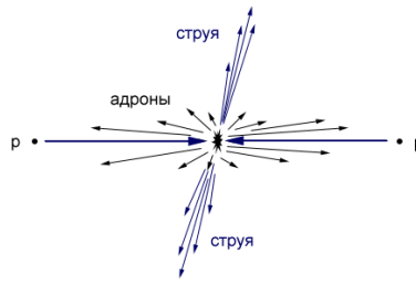
Рис.1 Схематичное представление процесса множественного рождения адронов [2].
