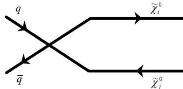
Рис,4 Диаграмма Фейнмана для u -канала подпроцесса столкновения двух кварков д) u канал с поляризацией
