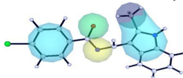
Şəkil 1 Bakterial qlükuronidazanın effektiv inhibitorlarının ümumiləşdirilmiş modeli
