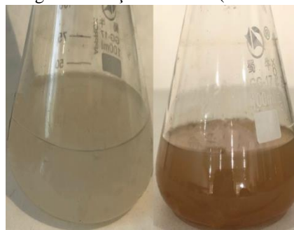
Şəkil 2. Ş 2 ştamının biokütləsində \text{AgNO}_3 əmələ gəlməsi müşahidə olunur (7-ci sutkada)
