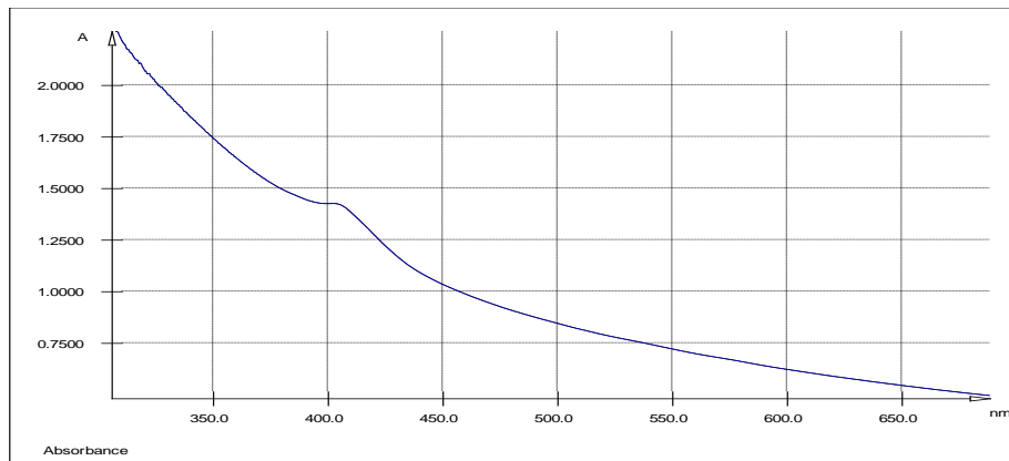
Şəkil 1. UV – VİS spektrofotometrik analiz, sintetik qidalı mühitdə 400-450 nm udulma halı
