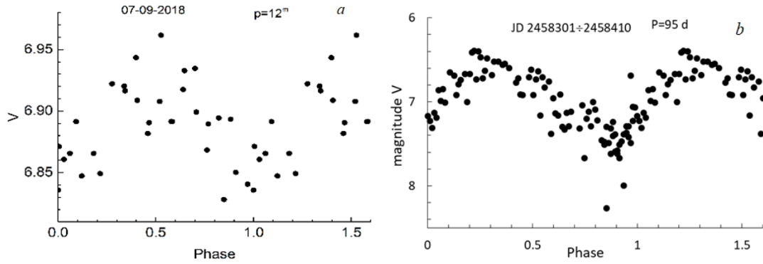
Şəkil 3. CH Cyg-nin V filtrində parlaqlığın faza diaqramları. a - 07-09-2018 tarixi, P=12 dəqiqə; b - 30-06 ÷ 18-10-2018 aralığı, P = 95 gün.
