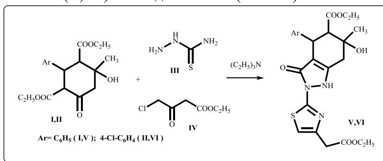
Схема 4. Синтез биядерных гетероциклических систем – этил-2-(4-(2-этокси-2-оксоэтил)тиазол-2-ил)-6-гидрокси-6-метил-3-оксо-4-арил-2,3,4,5,6,7-гексагидро-1H-индазол-5-карбоксилатов ( V , VI )
