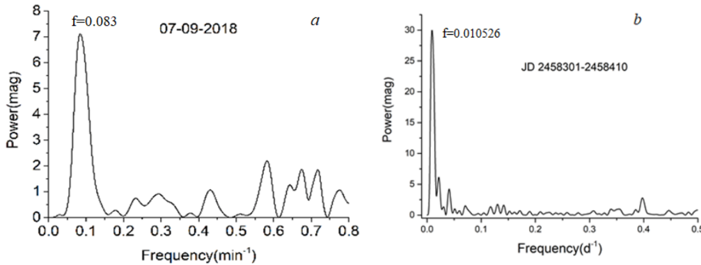
Şəkil 2. V qiymətlər massivinə görə güc spektri. a - 07-09- 2018 tarixi üçün 0÷0.8 tezlik intervalında güc spektri, b - 30-06 ÷ 18-10-2018 aralığı üçün 0÷0.5 tezlik intervalında güc spektri.
