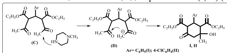
Схема 3. Внутримолекулярная кетонизация с образованием диэтил-2-арил-4-гидрокси-4-метил-6-оксоциклогексан-1,3-дикарбоксилаты (I, II)
