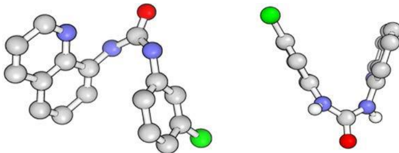
Şəkil 2. Energetik cəhətdən səmərəli olan II-4 inhibitorunun U-şəkilli konformeru
