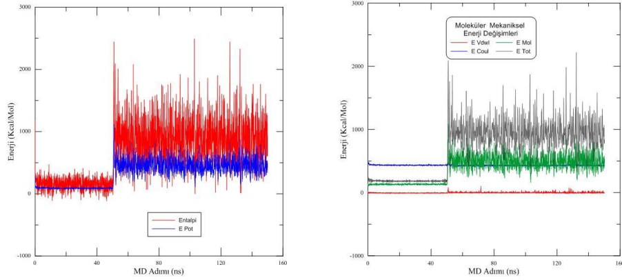
Şekil 2. Simülasyon adım sayısına göre enerji değişimleri
