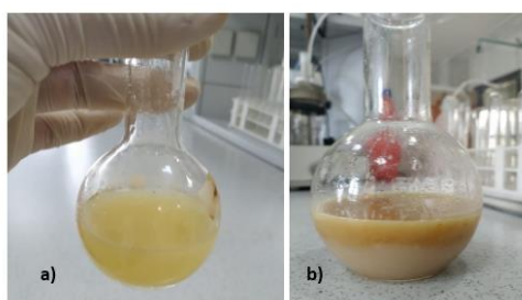
Şəkil2. A) I mərhələ- günəbaxan yağından Qliserol mürəkkəb efinin (monoqliserid), yəni aralıq məhsulun sintezi, b) II mərhələ- Qliserol mürəkkəb efinə neytral ikili səthi aktiv maddənin (GS) sintezi.
