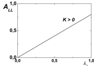
Рис.5 Зависимость коэффициента асимметрии от поляризации \lambda_2 .
