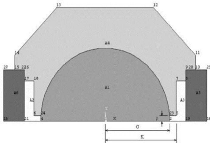
Şəkil 6. Maqnit avadanlığın forması
