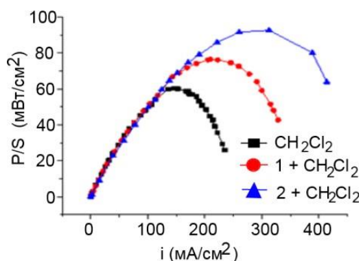
Şəkil 4. Anod mühitində 10 µL CH 2 Cl 2 -yə CH 2 Cl 2 -də 1 və 2 komplekslərinin 5,10-4 mol L məhlulunu əlavə etdikdən sonra 4,0 mQ/sm 2 Pt/Nf MEA olan yanacaq elementinin diaqnostik əyrisi.
