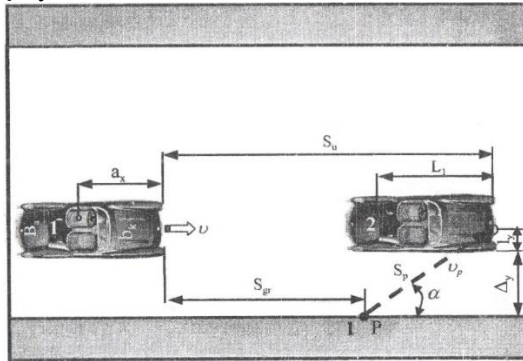
Şəkil 1. Nəqliyyat vasitəsinin qabaq hissəsi ilə iti bucaq istiqamətində hərəkət edən piyadanın vurulması sxemi
