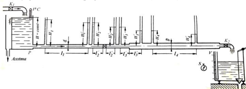
Şəkil 1. Hidravlik müqavimət əmsallarının eksperimental tədqiqat qurğusu
